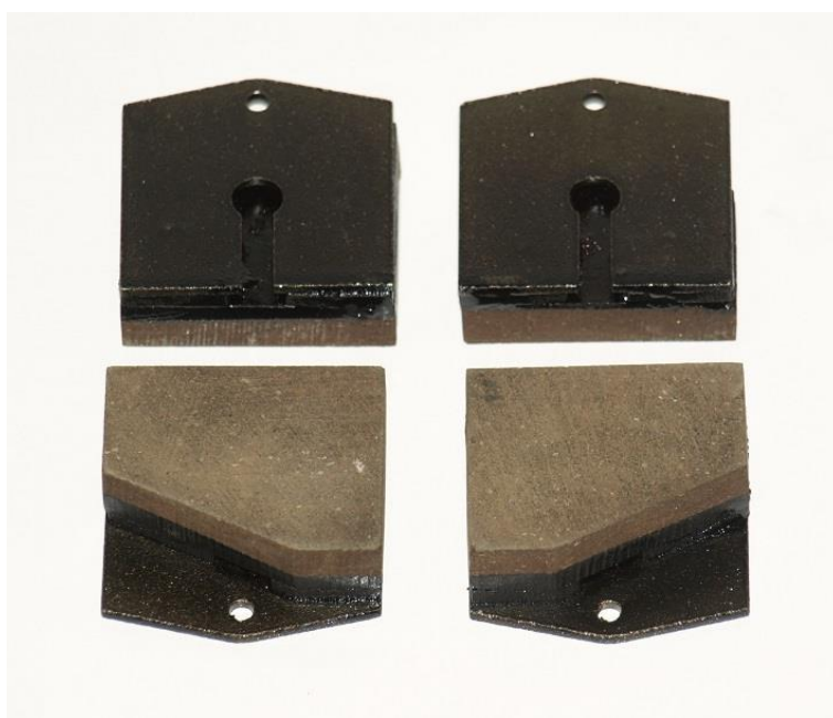
Brzdové segmenty pro ruční brzdu TATRA 603
